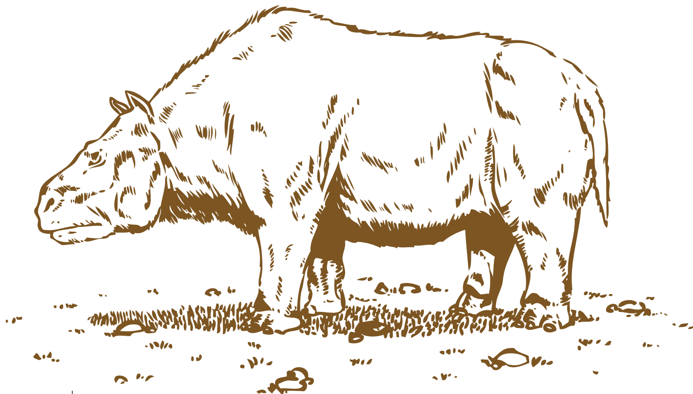
Toxodon platensis
